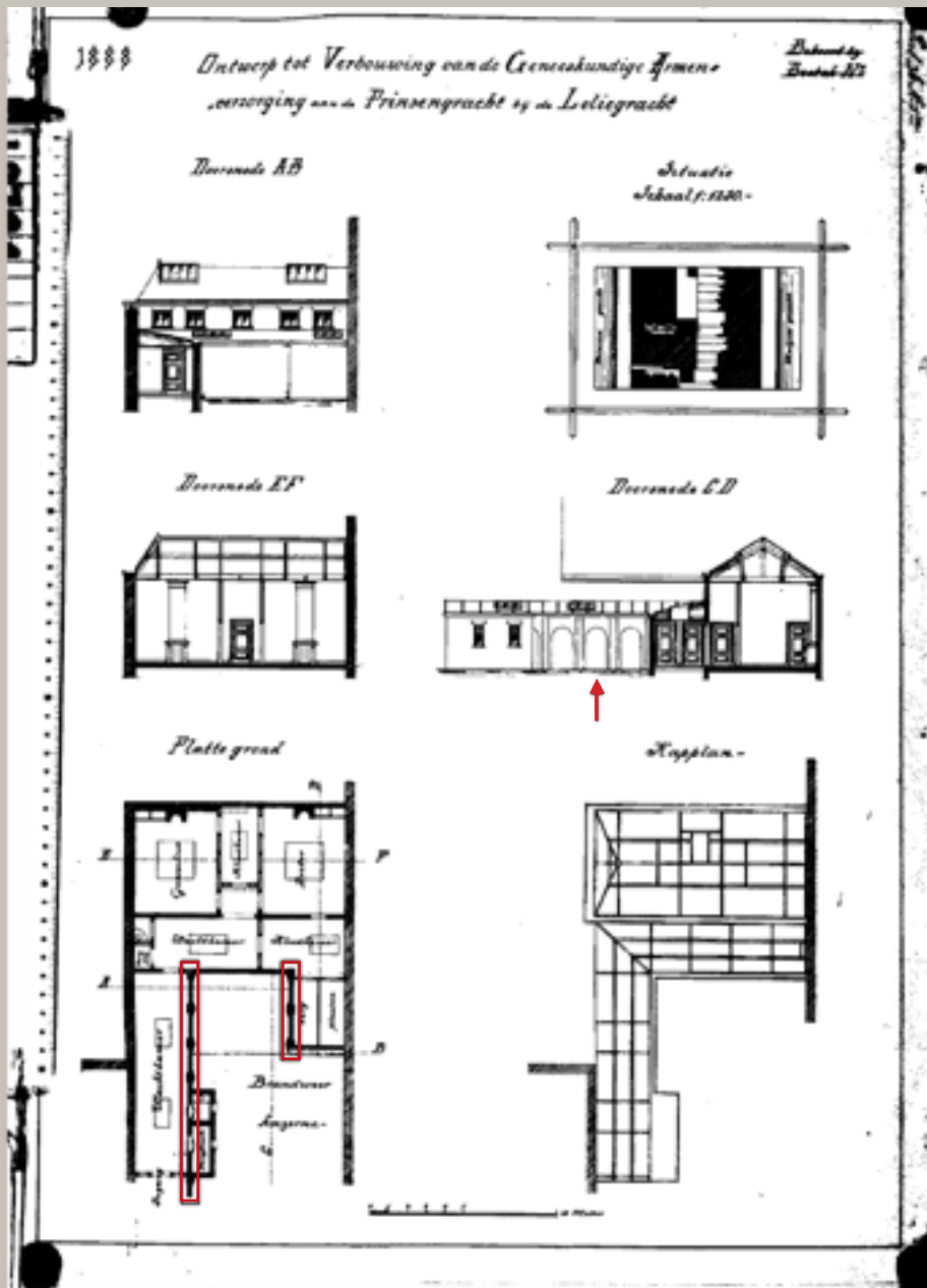
Bouwtekening uit 1888, die is gemaakt ten behoeve van de verbouwing van het inmiddels gesloopte achterhuis (voormalig inschrijfkantoor). Op deze tekening zijn de zeventiende-eeuwse galerijbogen nog duidelijk zichtbaar, zie rode markering (Stadsarchief Amsterdam, archief 10057, inv.nr. 18704)
